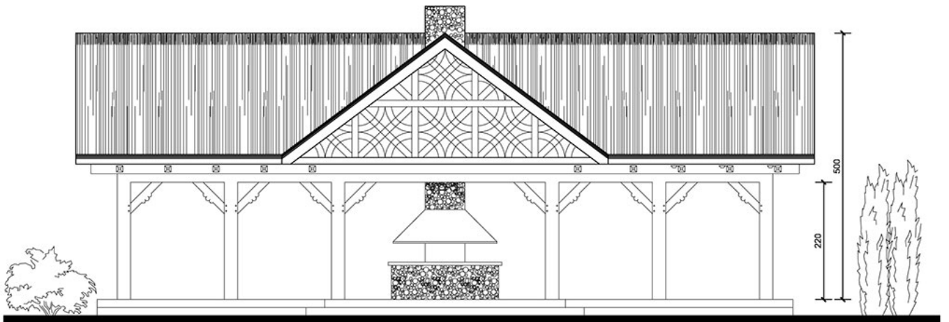
ELEWACJA FRONTOWA
