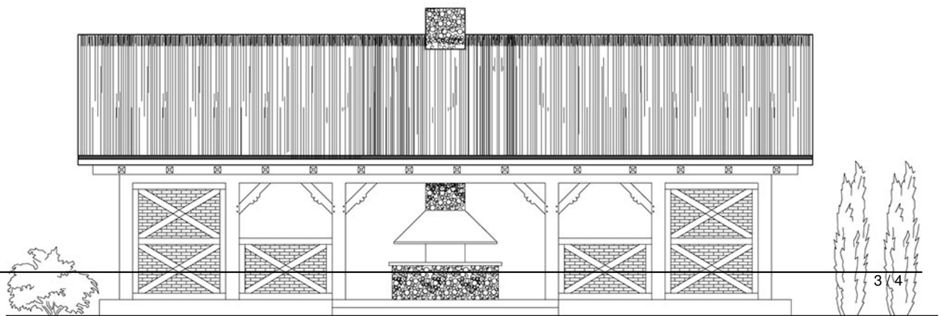
ELEWACJA TYLNA
